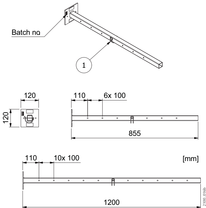
Bild 10. Teleskoparm
