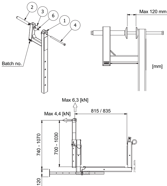
Bild 4. Hängbryggetving
