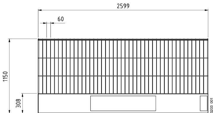
Bild 17. Räckesnät Stål
