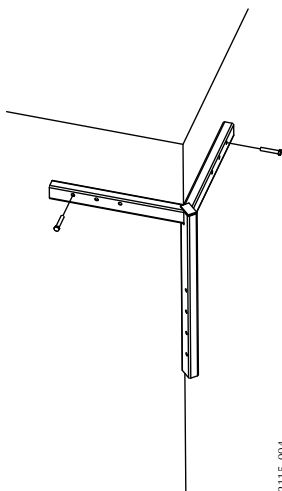
Bild 35. Montering av Hörnbrygga Infästning
