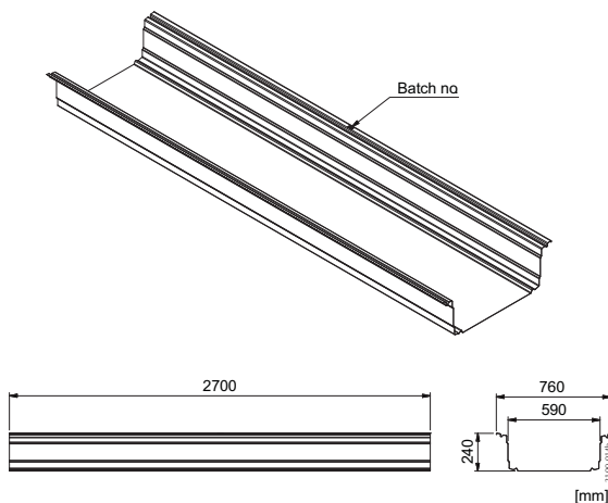
Bild 9. Gångplåt
